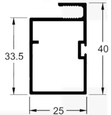
P227 / 25549 Peso: 0,509 kg/m
