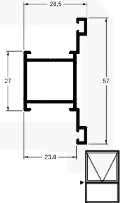
SK085 / SU085 Peso: 0,501 kg/m Travessa MAXIMAR
