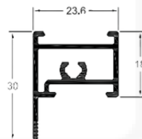
SK082 / SU082 Peso: 0,382 kg/m FolhaTravessa MAXIMAIR
