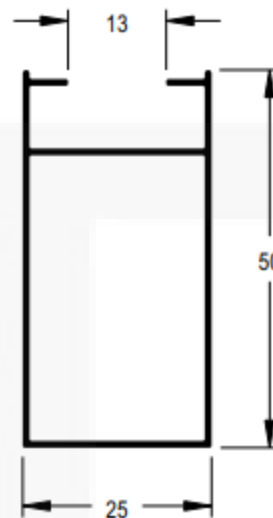
A4A231 Peso: 0,216 kg/m
