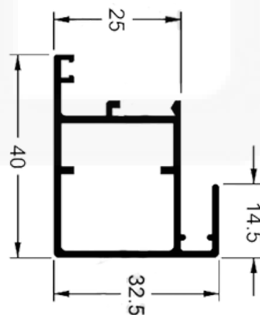
P151 / 25568 Peso: 0,585 kg/m
