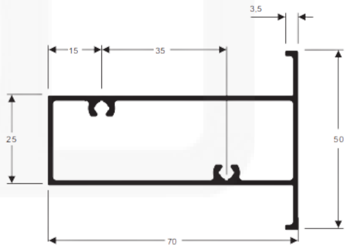
P274 Peso: 0,856 kg/m
