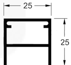
A056 / 25571 Peso: 0,404 kg/m
