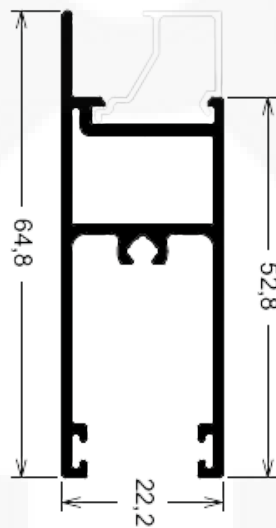
SK272 / SU272 Peso: 0,452 kg/m Marco Trilho Inferior Portas
