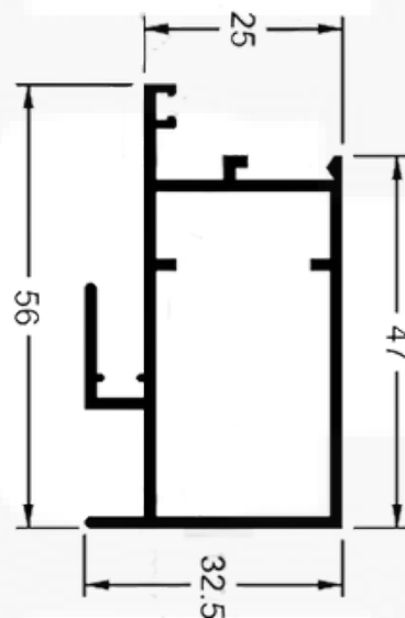
P151 / 25568 Peso: 0,585 kg/m
