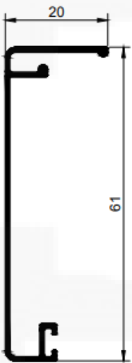
E512A Peso: 0,263 kg/m
