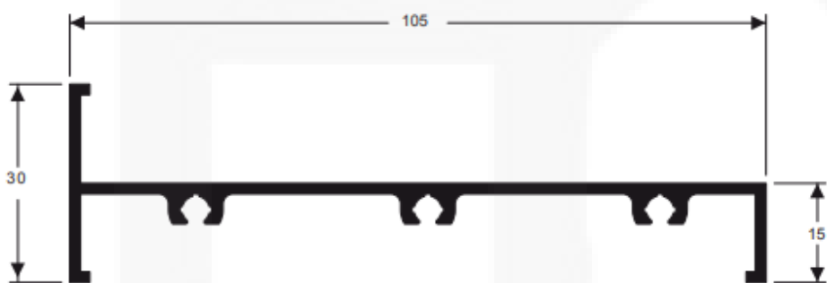
Y260 Peso: 0,718 kg/m
