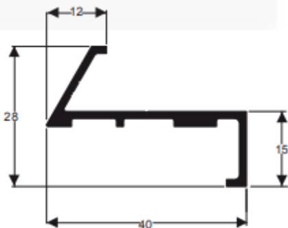
Z033 Peso: 0,315 kg/m
