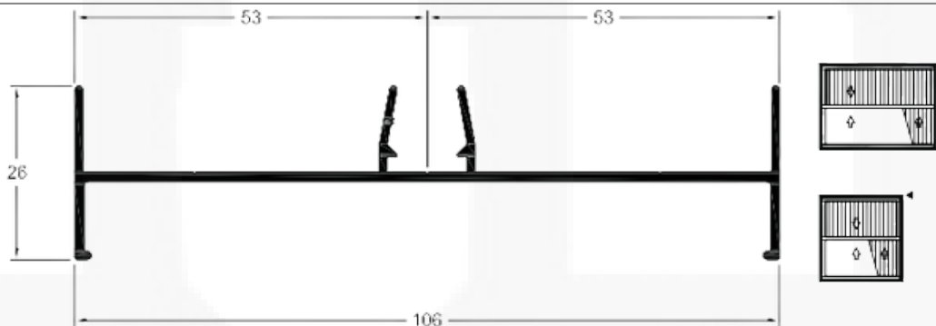
SK014 / SU014 Peso: 0,676 kg/m Marco Montante Lateral Janelas e Portas
