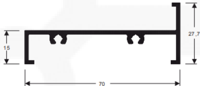
Z175 Peso: 0,509 kg/m
