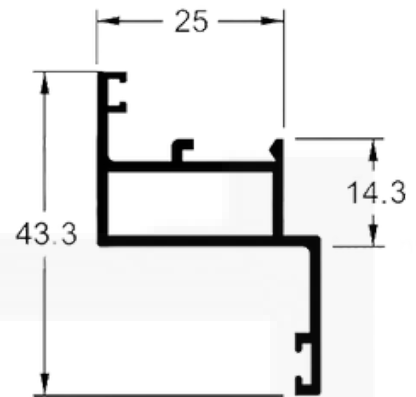
P145 / 25572 Peso: 0,466 kg/m
