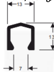
U681 Peso: 0,133 kg/m
