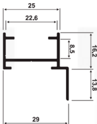
SK071 / SU071 Peso: 0,255 kg/m
