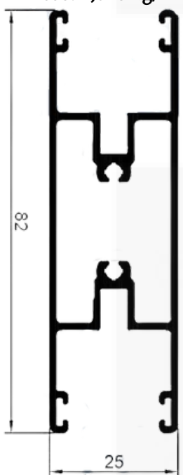
MN027 Peso: 1,018 kg/m
