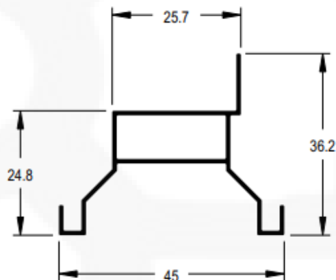
A4A055 Peso: 0,319 kg/m
