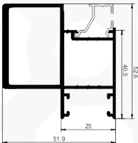
SK044 / SU044 Peso: 0,972 kg/m
