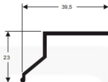
L332 Peso: 0,198 kg/m
