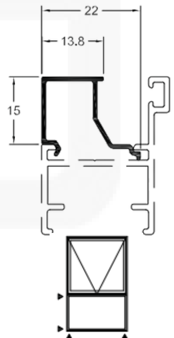
SK103 / SU103 Peso: 0,141 kg/m Baguete Fixo MAXIMAR
