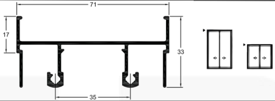
SK001 / SU001 Peso: 0,756 kg/m Marco Trilho Superior Janelas e Portas
