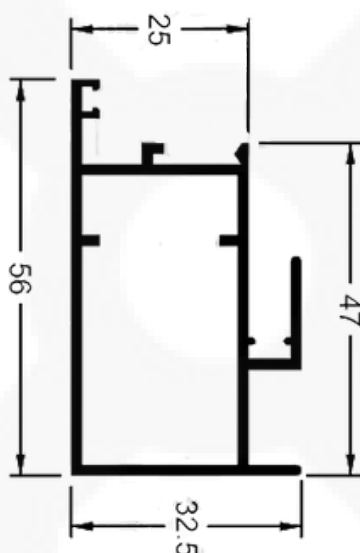
P152 / 25569 Peso: 0,463 kg/m
