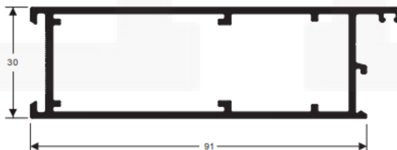
P264 Peso: 1,093 kg/m
