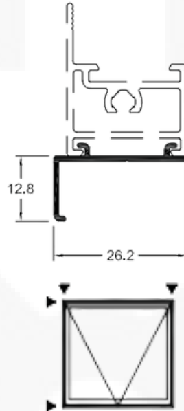
SK084 / SU084 Peso: 0,125 kg/m Pingadeira MAXIMAR
