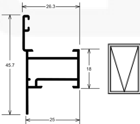
SK200 / SU200 Peso: 0,381 kg/m
