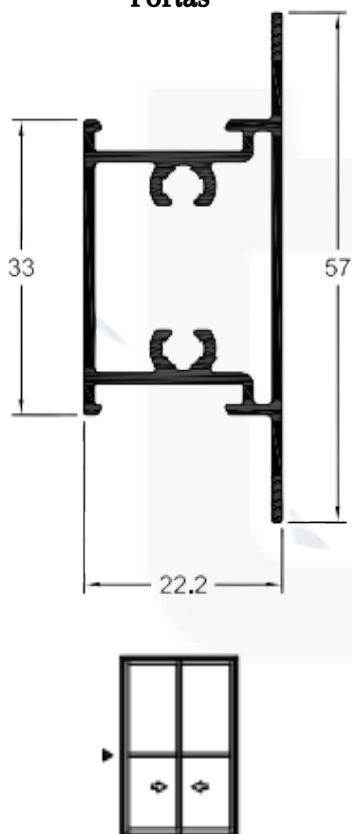
SK227 / SU227 Peso: 0,551 kg/m Travessa Intermediária Portas
