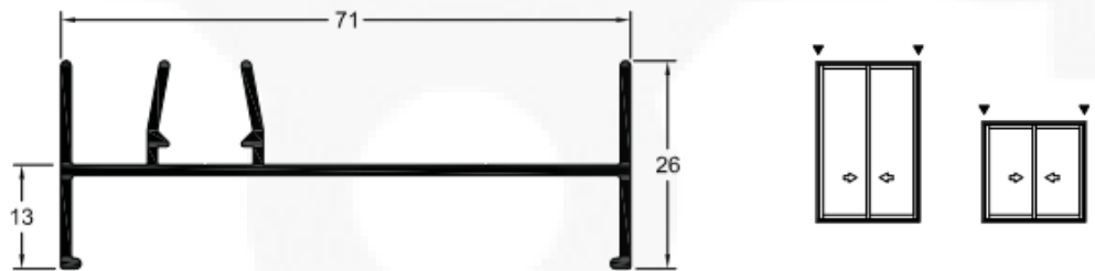
SK003 / SU003 Peso: 0,526 kg/m Marco Montante Lateral Janelas e Portas
