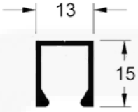
U425 / 25662 Peso: 0,157 kg/m
