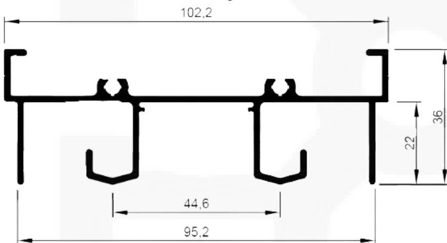
LG044 / AK300 Peso: 1,245 kg/m
