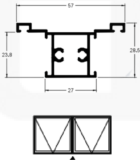
SK086 / SU086 Peso: 0,539 kg/m Montante Lateral MAXIMAR
