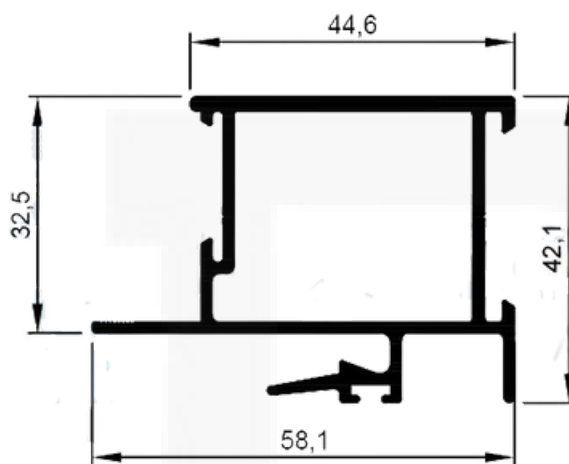
LG048 / AK409 Peso: 0,966 kg/m
