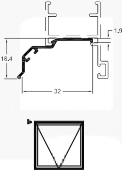
SK083 / SU083 Peso: 0,149 kg/m Pingadeira MAXIMAR
