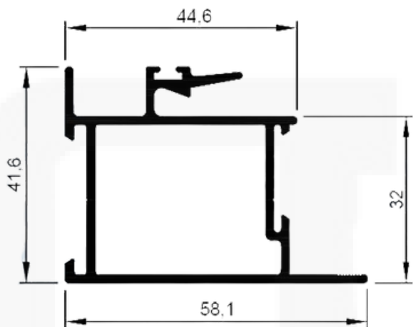
LG049 / AK408 Peso: 0,906 kg/m
