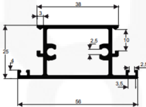
P319 / 25522 Peso: 0,721 kg/m
