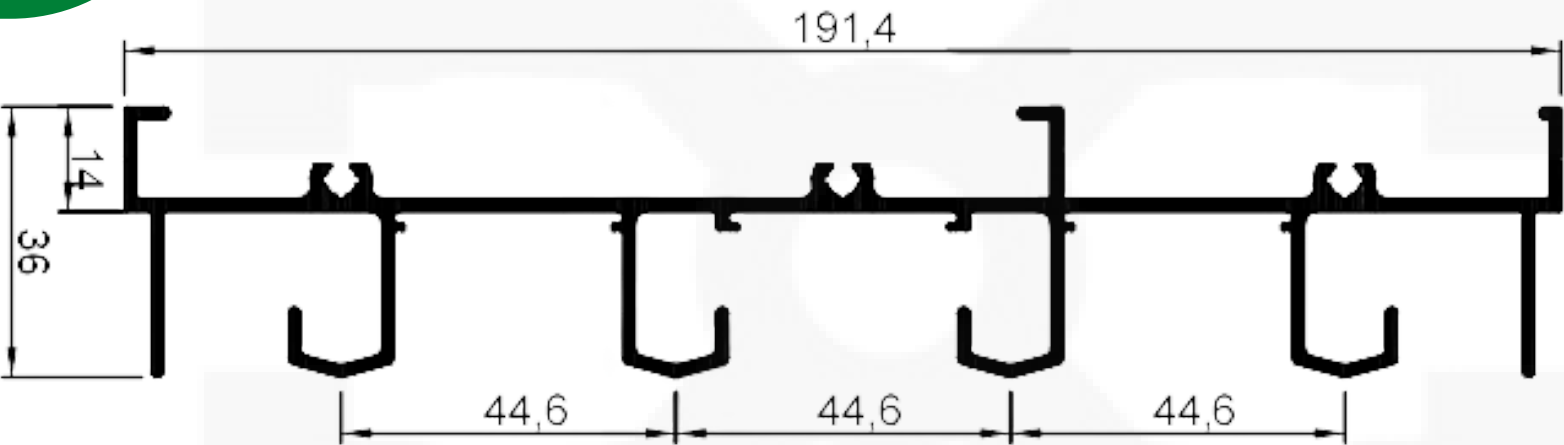
AK506 Peso: 2,273 kg/m
