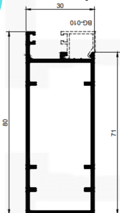
P358 / 30033 Peso: 0,944 kg/m
