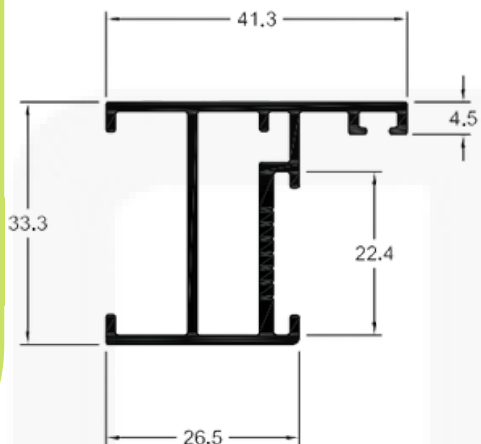
SK043 / SU043 Peso: 0,976 kg/m
