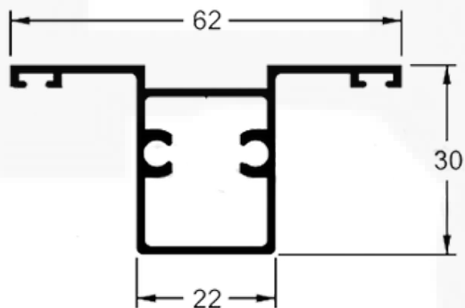
P574 / 25669 Peso: 0,631 kg/m
