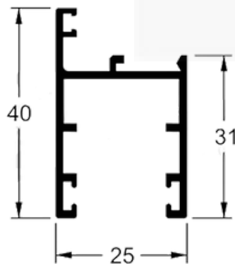
Y195 / 25565 Peso: 0,474 kg/m
