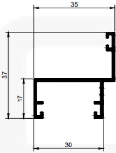
Y140 / 30054 Peso: 0,352 kg/m
