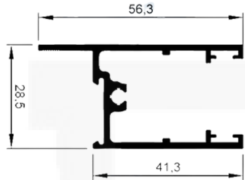
LG006 / AK402 Peso: 0,676 kg/m
