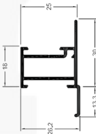
SK081 / SU081 Peso: 0.406 kg/m
