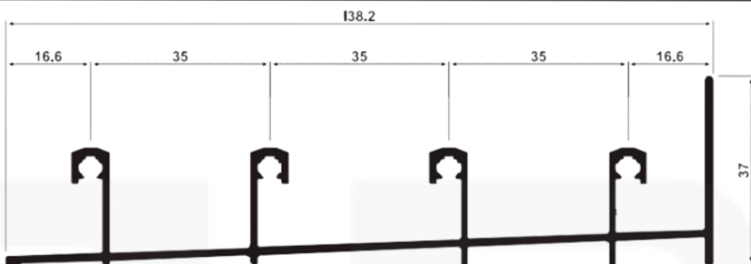
SK222 / SU222 Peso: 1,182 Soleira Porta Balcão
