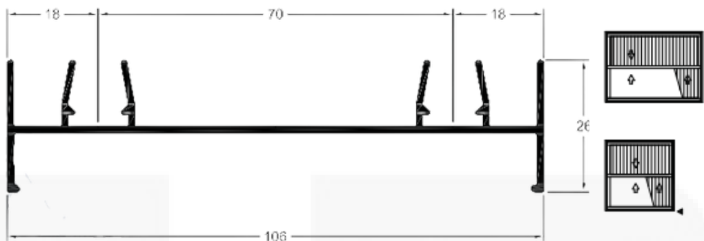
SK013 / SU013 Peso: 0,775 kg/m Marco Montante Lateral Janelas e Portas
