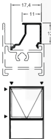
SK102 / SU102 Peso: 0,111 kg/m Baguete MAXIMAR
