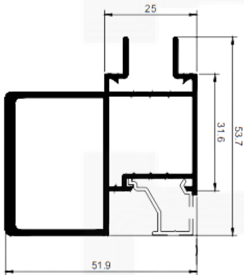
SK043 / SU043 Peso: 0,976 kg/m
