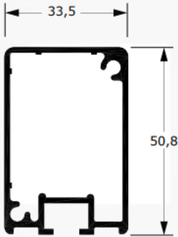
78088 Peso: 0,858 kg/m
