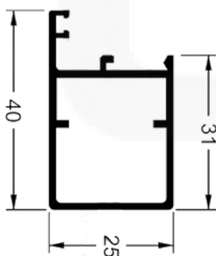
P140 / 25570 Peso: 0,504 kg/m
