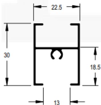
A4A057 Peso: 0,281 kg/m
