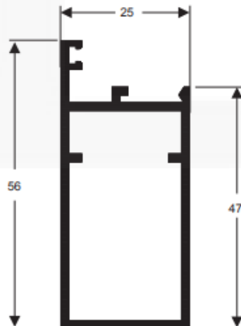
P318 Peso: 0,578 kg/m
