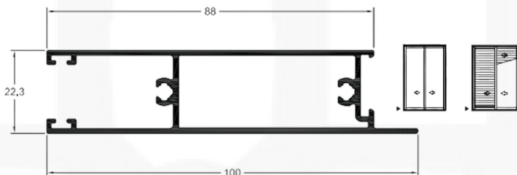
SK228 / SU228 Peso: 0,667 kg/m Marco Trilho Inferior Portas
