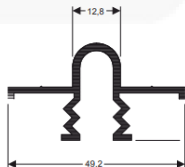
E364 Peso: 0,405 kg/m
