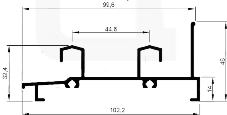
LG047 / AK328 Peso: 1,133 kg/m
