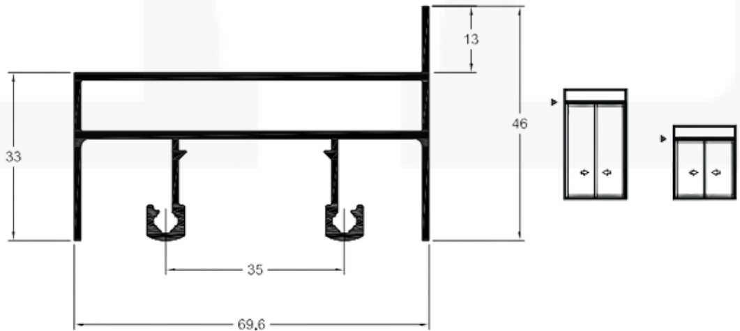
SK005 / SU005 Peso: 1,108 kg/m Travessa Bandeira Janelas e Portas
