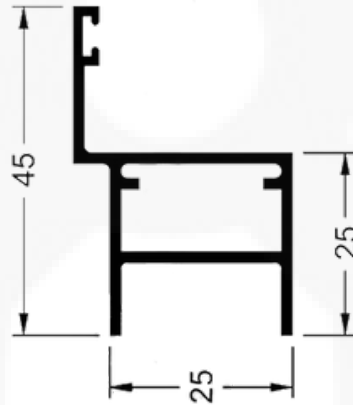
P155 / 25522 Peso: 0,526 kg/m
