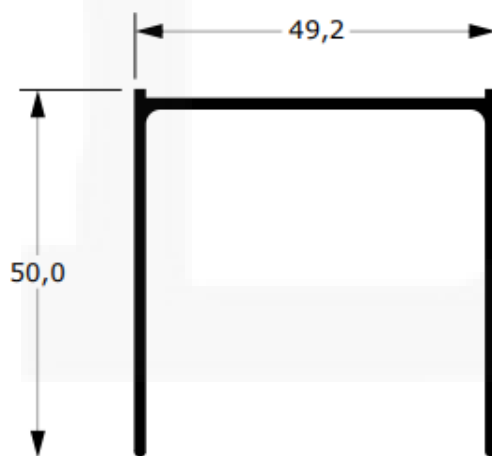
39498 Peso: 0,636 kg/m
