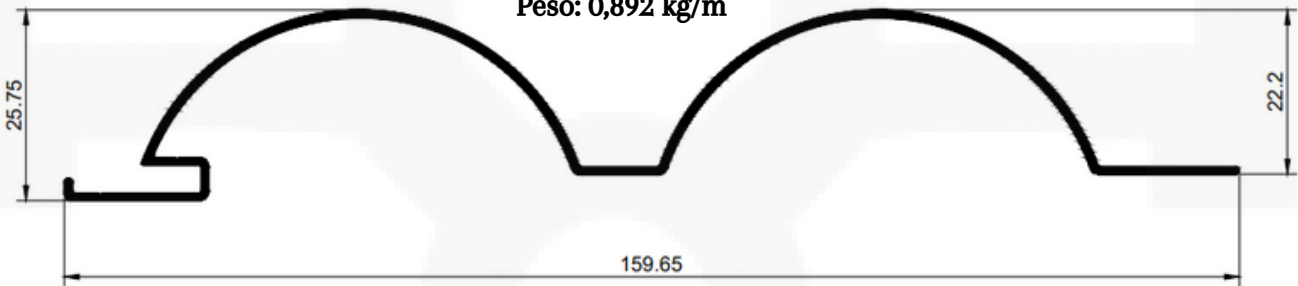
19575 Peso: 0,892 kg/m
