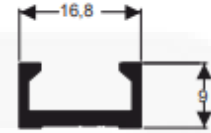
U683 Peso: 0,154 kg/m
