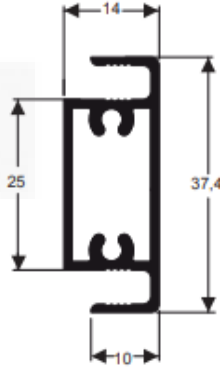
P056 Peso: 0,405 kg/m
