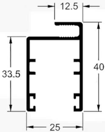
Y312 / 25551 Peso: 0,488 kg/m
