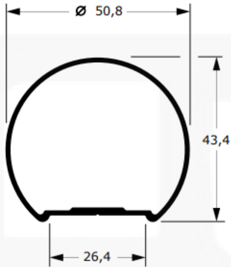
78260 Peso: 0,660 kg/m
