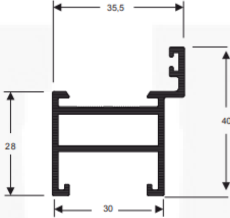
P273 Peso: 0,612 kg/m
