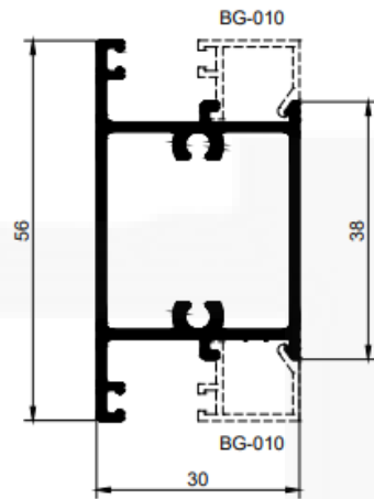
P078 / 30025 Peso: 0,718 kg/m
