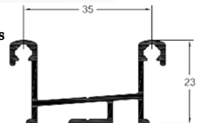
SK272 / SU272 Peso: 0,452 kg/m Marco Trilho Inferior Portas
