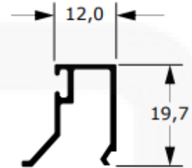
39077 Peso: 0,179 kg/m
