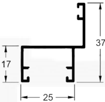
Y126 / 25556 Peso: 0,333 kg/m
