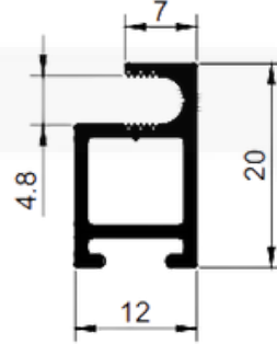
A058 Peso: 0,206 kg/m
