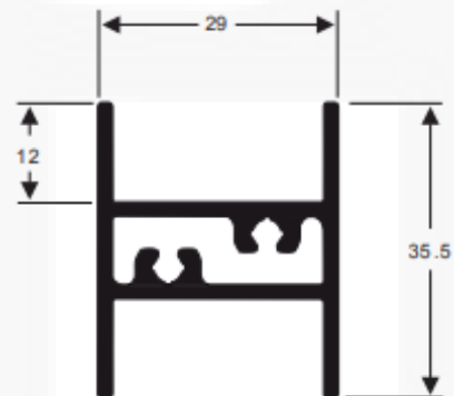
A084 Peso: 0,587 kg/m
