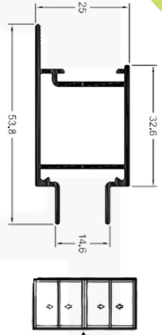
SK120 / SU120 Peso: 0,482 kg/m Montante Folha
