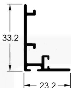
L498 / 25696 Peso: 0,271 kg/m
