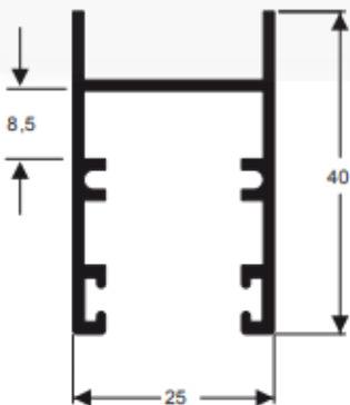
I122 Peso: 0,461kg/m
