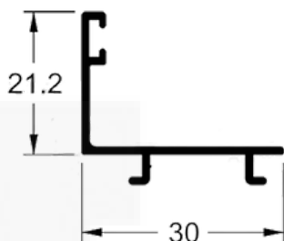
L383 / 25574 Peso: 0,222 kg/m
