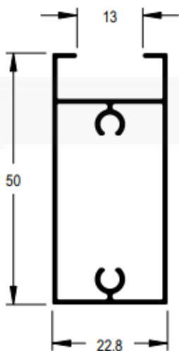
A4A230 Peso: 0,437 kg/m
