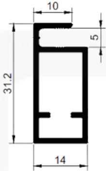
P027 Peso: 0,306 kg/m
