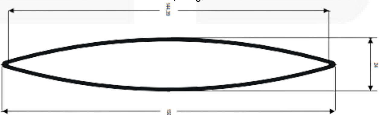
D053 Peso: 1,230 kg/m
