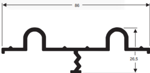
E365 Peso: 0,683 kg/m
