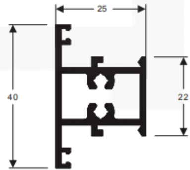
P153 Peso: 0,547 kg/m
