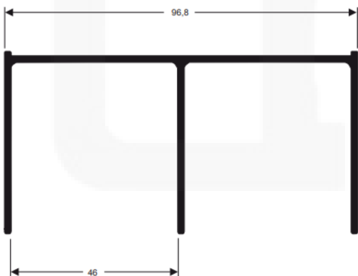
E363 Peso: 0,984 kg/m
