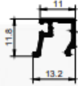
U522 / BG001 Peso: 0,103 kg/m
