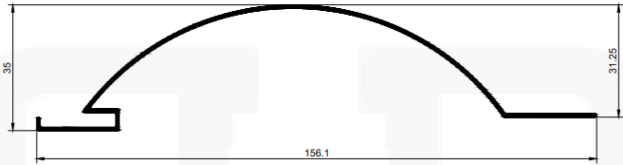
19505 Peso: 0,535 kg/m
