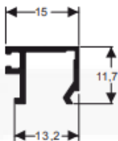
U482 / BG010 Peso: 0,100 kg/m
