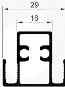
P256 / 25550 Peso: 0,496 kg/m
